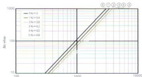
Потери напора на смесительном узле
